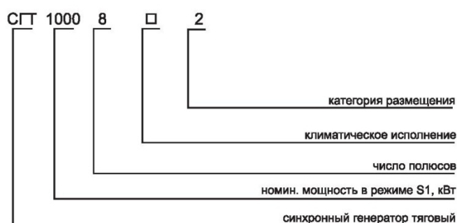
Структура условного обозначения генераторов синхронных типа СГТ-1000
