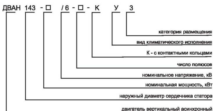
Структура условного обозначения двигателей типа ДВАН
