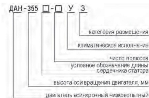
Структура условного обозначения двигателей типа ДАН
