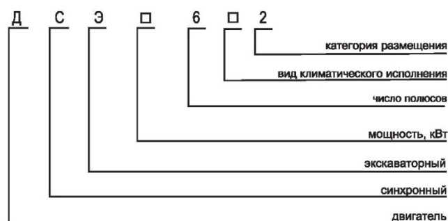
Структура условного обозначения двигателей серии ДСЭ-750, 630
